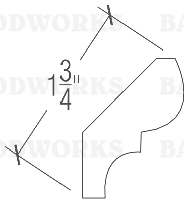
604A Bed Mould
